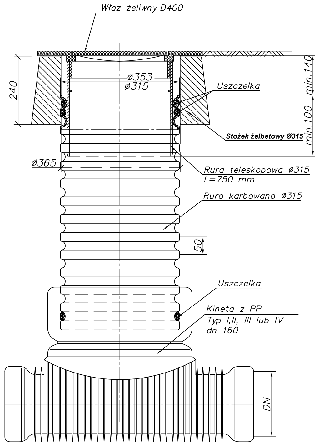
Studzienka inspekcyjna \varnothing 315 z rurą teleskopową
